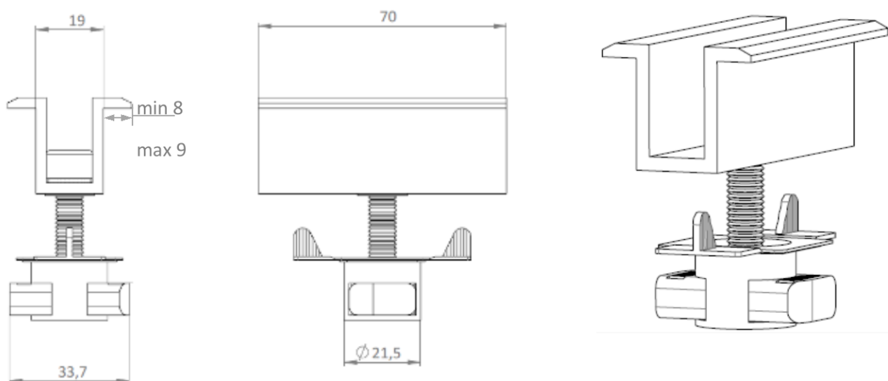
Figure 12 : Étrier intermédiaire
