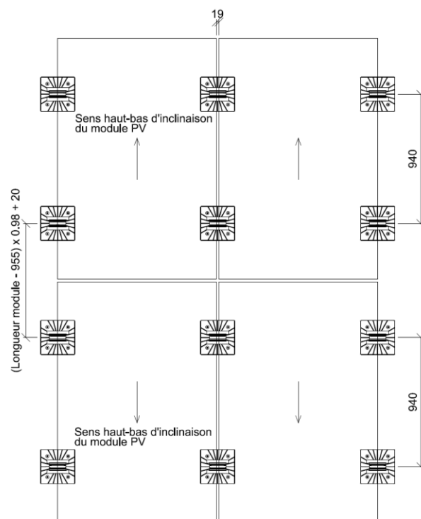
Figure 34 : Implantation des plots SOPRASOLAR FIX EVO avec modules photovoltaïques en inclinaison double shed – rehausse polymère 210 et réhausse aluminium 210
