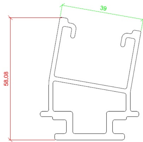
Figure 16 : Plan Réhausse 45 aluminium
