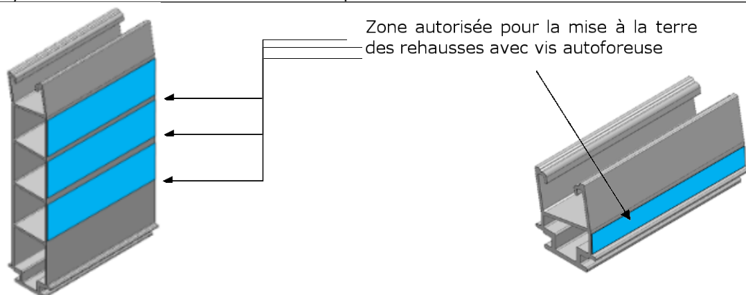
Localisation zone de perçage pour mise à la terre des rehausse Aluminium par vis autoperceuse (mise à la terre de la rehausse 200 &amp; 210 aluminium uniquement)
