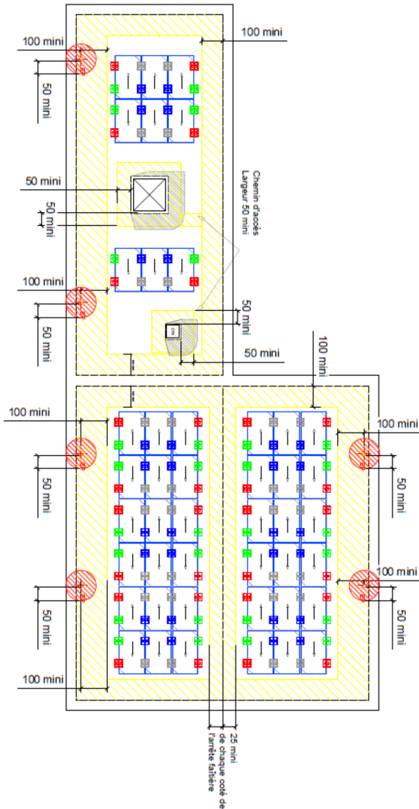
Figure 44 : Exemple calepinage et préparation de la toiture avec modules photovoltaïques inclinés en orientation double shed
