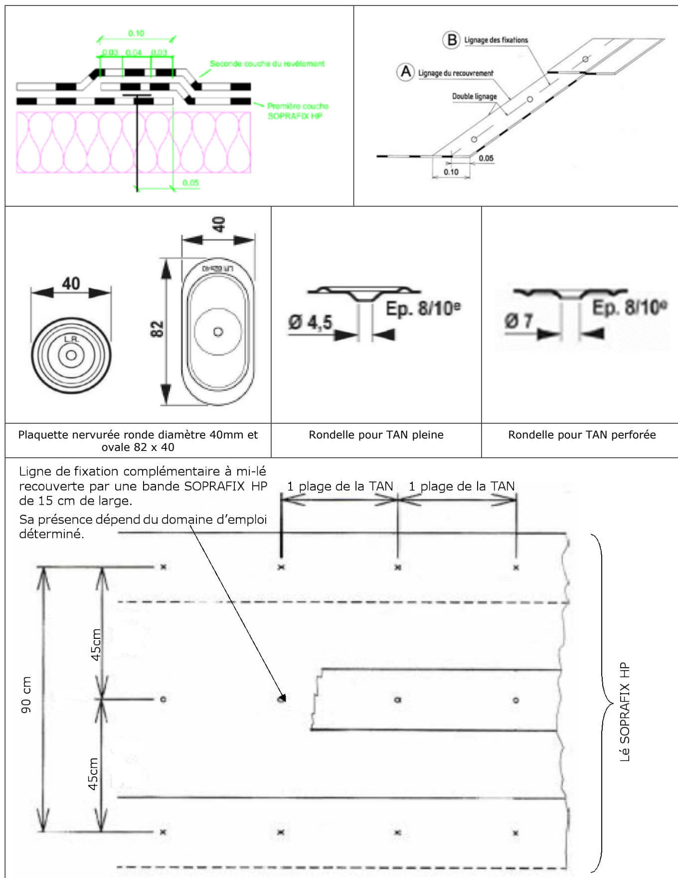
Figure 29 : Mise en œuvre du revêtement d'étanchéité avec première couche SOPRAPHIX HP et plaque de répartition
