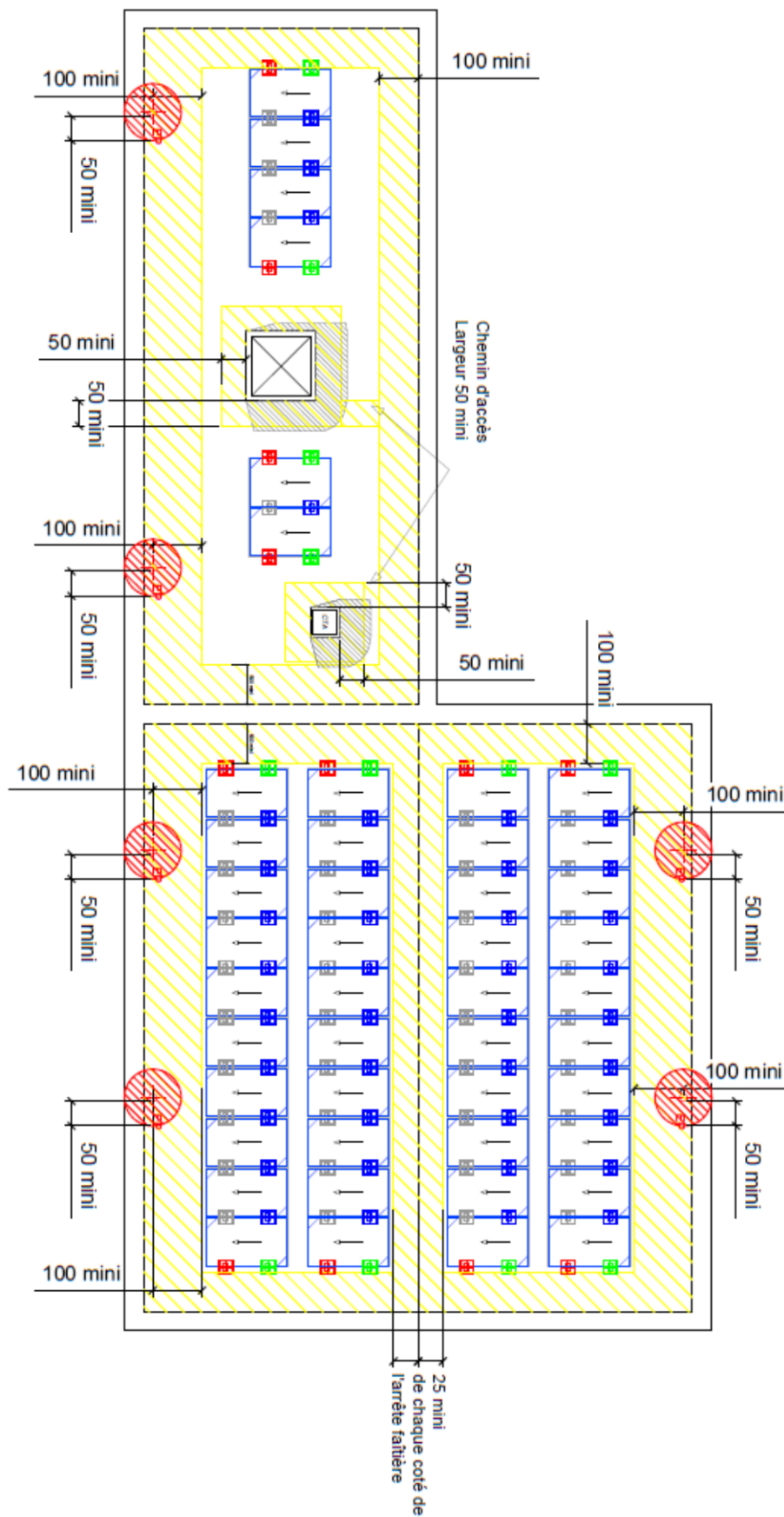
Figure 45 : Exemple calepinage et préparation de la toiture avec modules photovoltaïques inclinés en orientation simple shed
