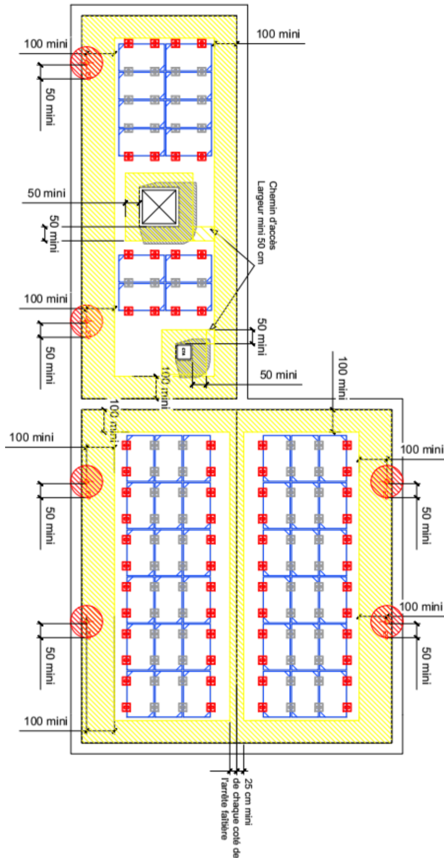
Figure 42 : Exemple calepinage standard (2 plots/grand côté du module) et préparation de la toiture en pose à plat
