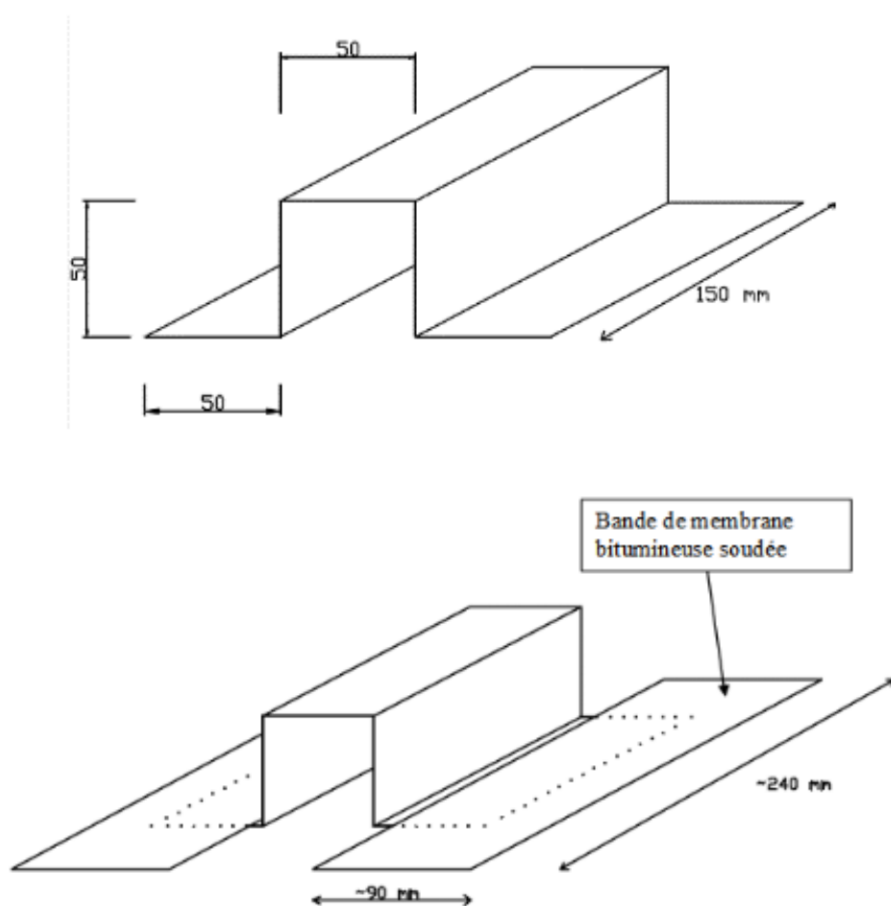
Figure 22 : Supports de chemin de câble par oméga
