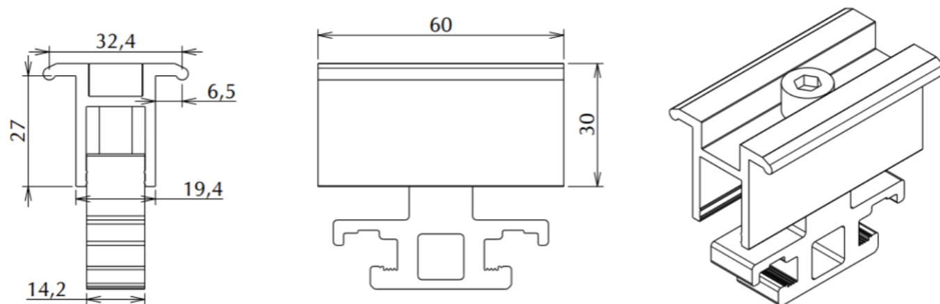
Figure 14 : Étrier universel STIB
