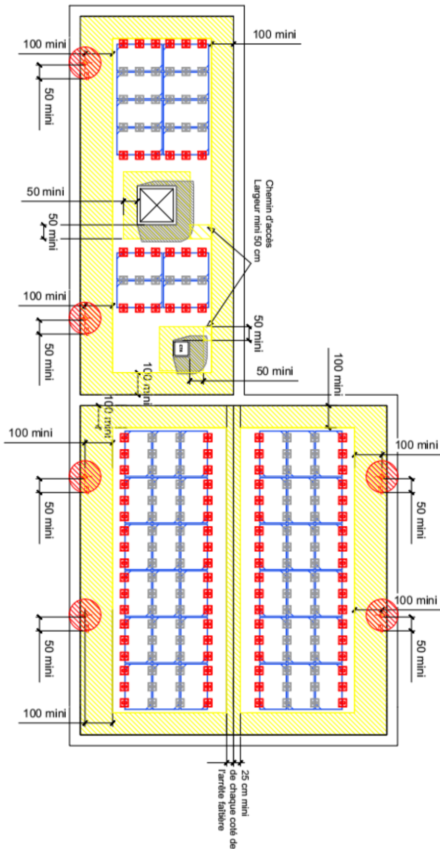
Figure 43 : Exemple calepinage standard (3 plots/grand côté du module) et préparation de la toiture en pose à plat
