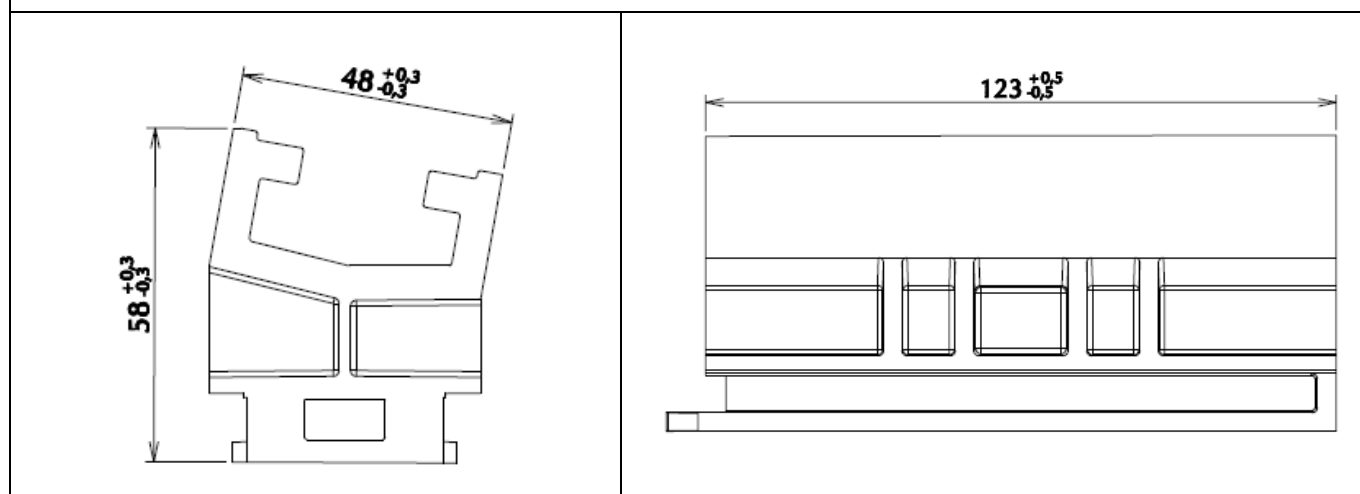
Figure 18 : Plan Réhausse 45 polymère
