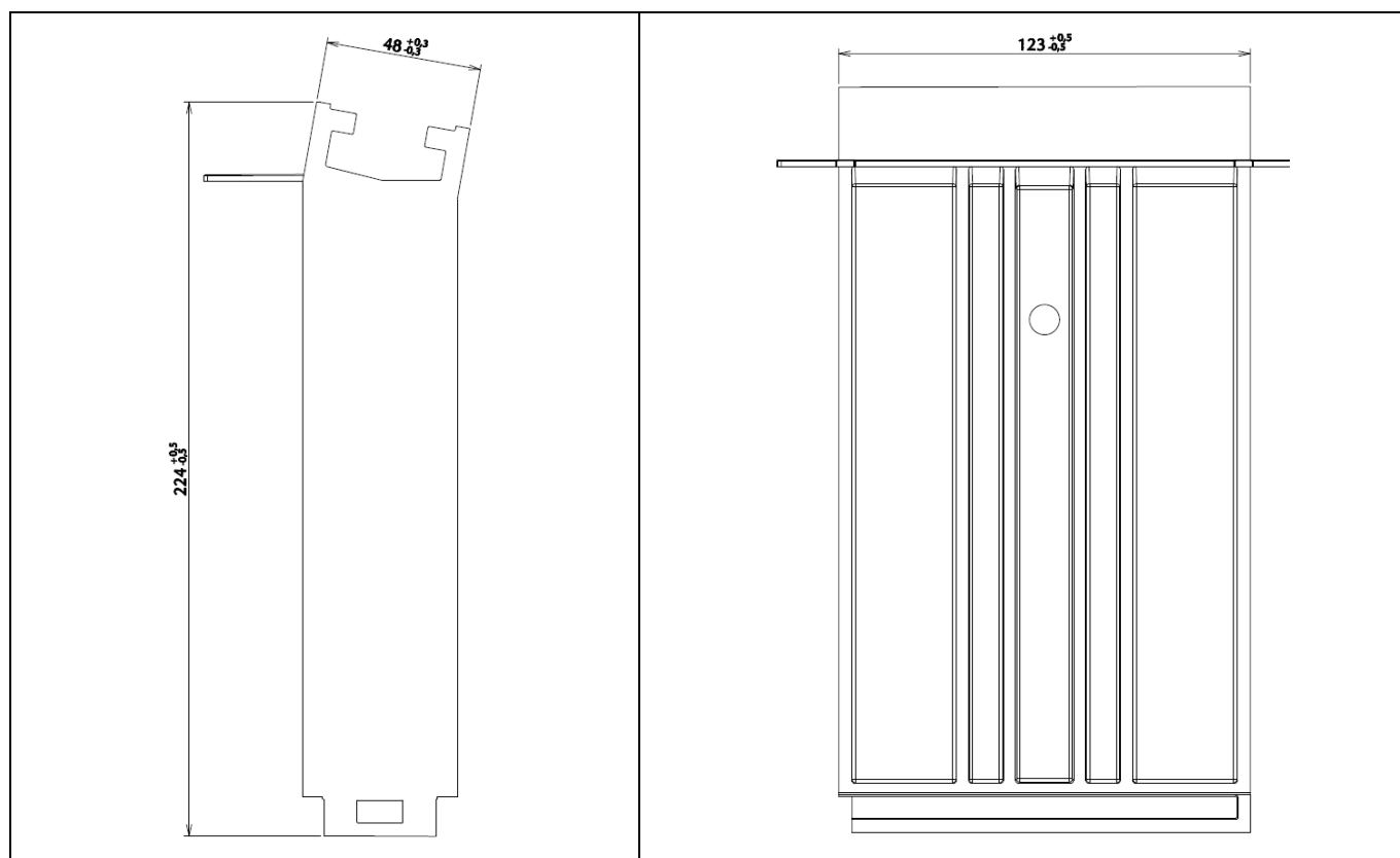
Figure 18 : Plan Réhausse 45 polymère
