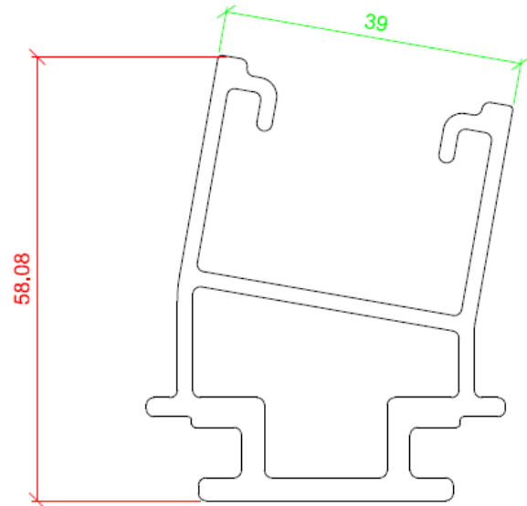
Figure 16 : Plan bloqueur de réhausse
