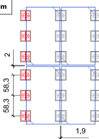
Figure 32 : Implantation des plots SOPRASOLAR FIX EVO PVC/TPO en calepinage densifié
