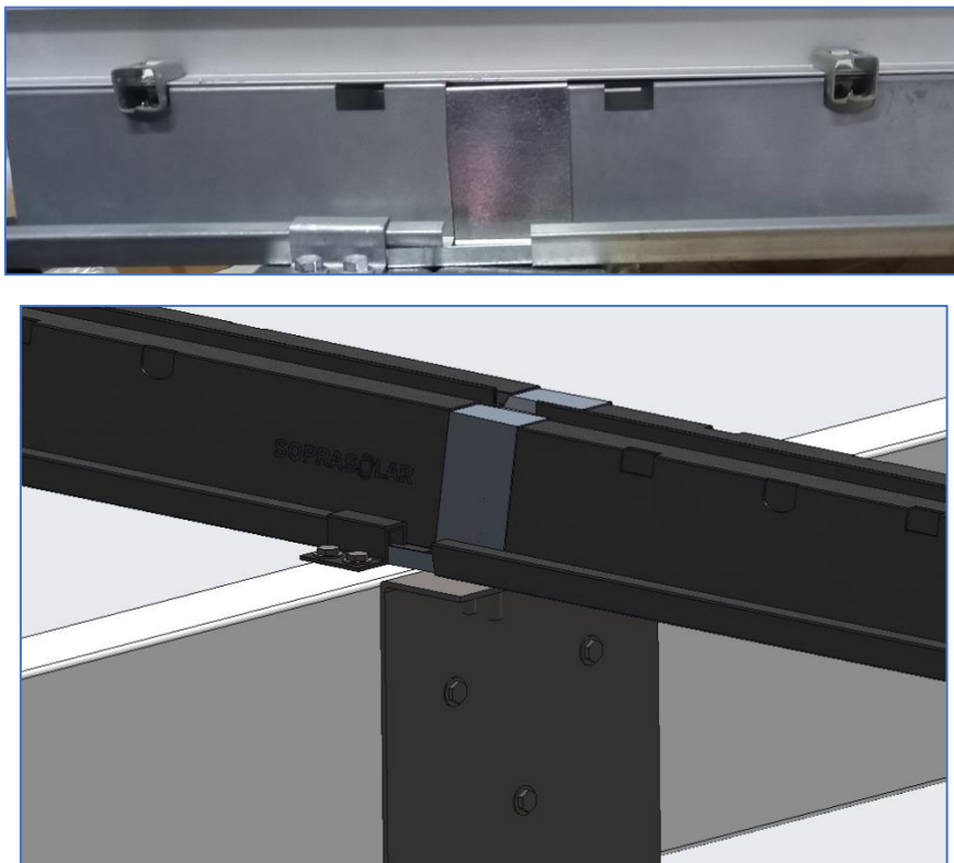
Figure 4 : Mise en œuvre de l'éclisse après fixation
