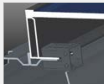
4 - Fixation des modules aux rails Soprasolar® Park avec le Soprasolar® Clips et raccordement électrique.
