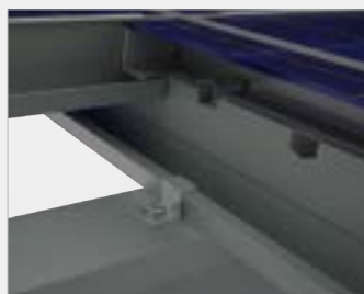
2 - Fixation des rails Soprasolar® Park aux pannes par crapauds.
